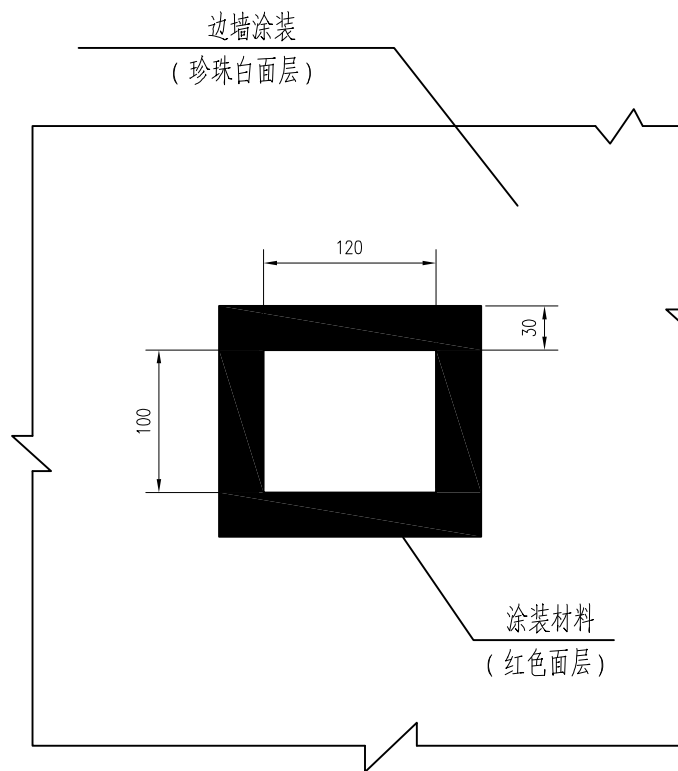
消防洞室I涂装立面图
