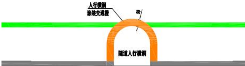
图 6 公路隧道人行横通道设计
