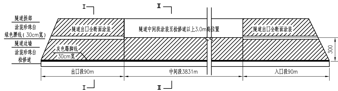
隧道左洞涂装立面图
