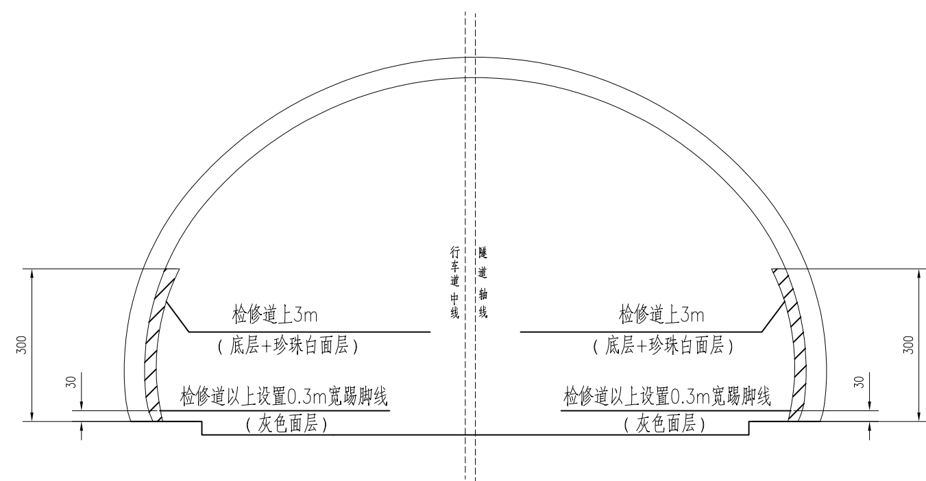
隧道洞壁涂装布置图
