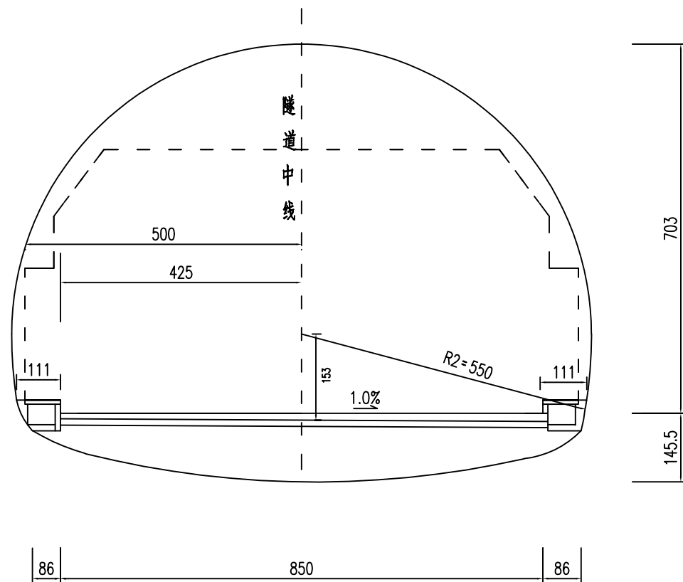
隧道衬砌内空断面图 1: 100
