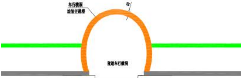
图 7 公路隧道车行横通道设计
