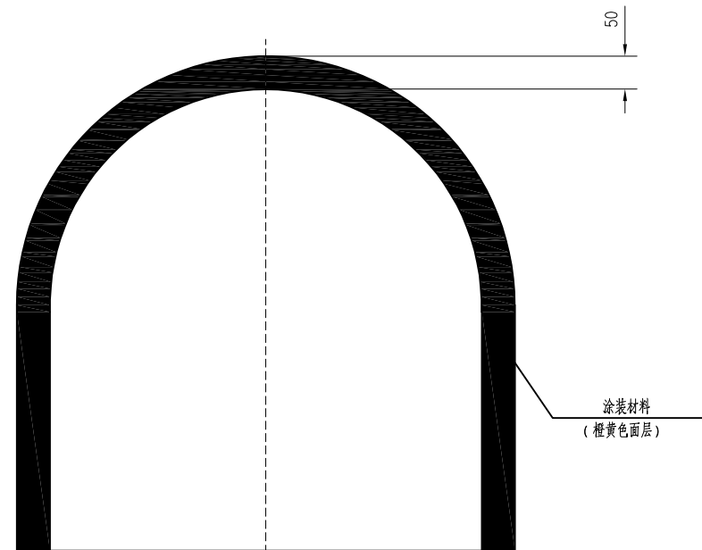
人行横洞涂装立面图 1:50
