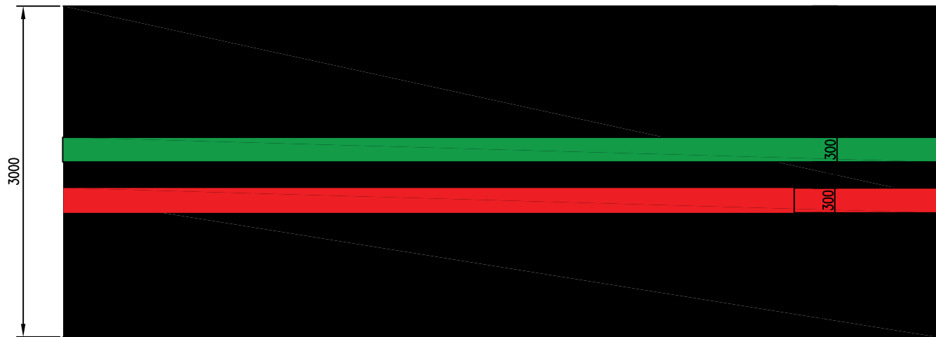
边墙3000mm范围喷涂白色布置图
