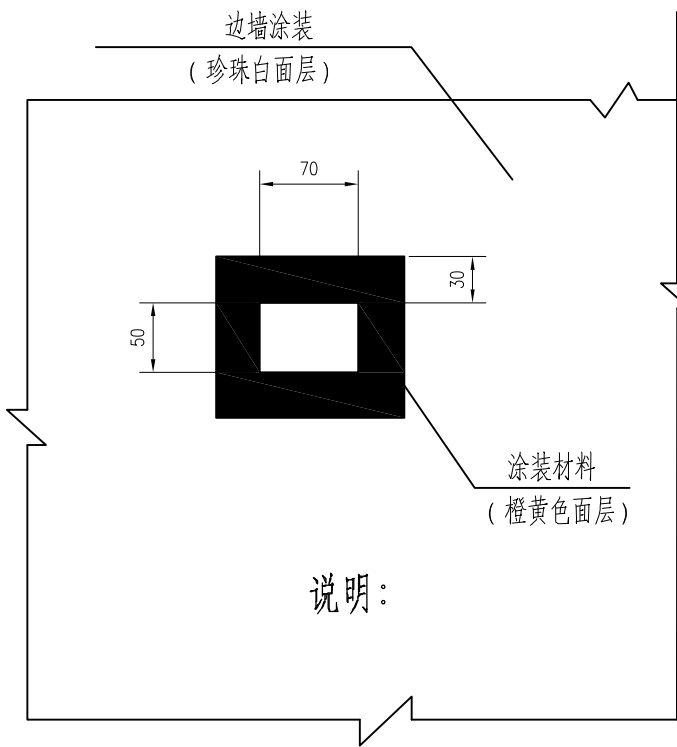
配电箱边框涂装立面图
