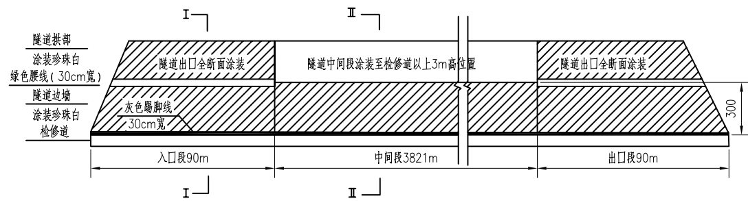
隧道右洞涂装立面图
