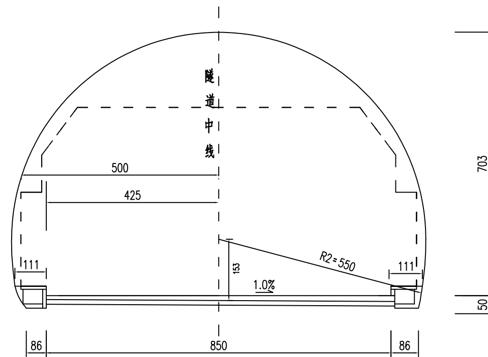
隧道衬砌内空断面图 1: 100
