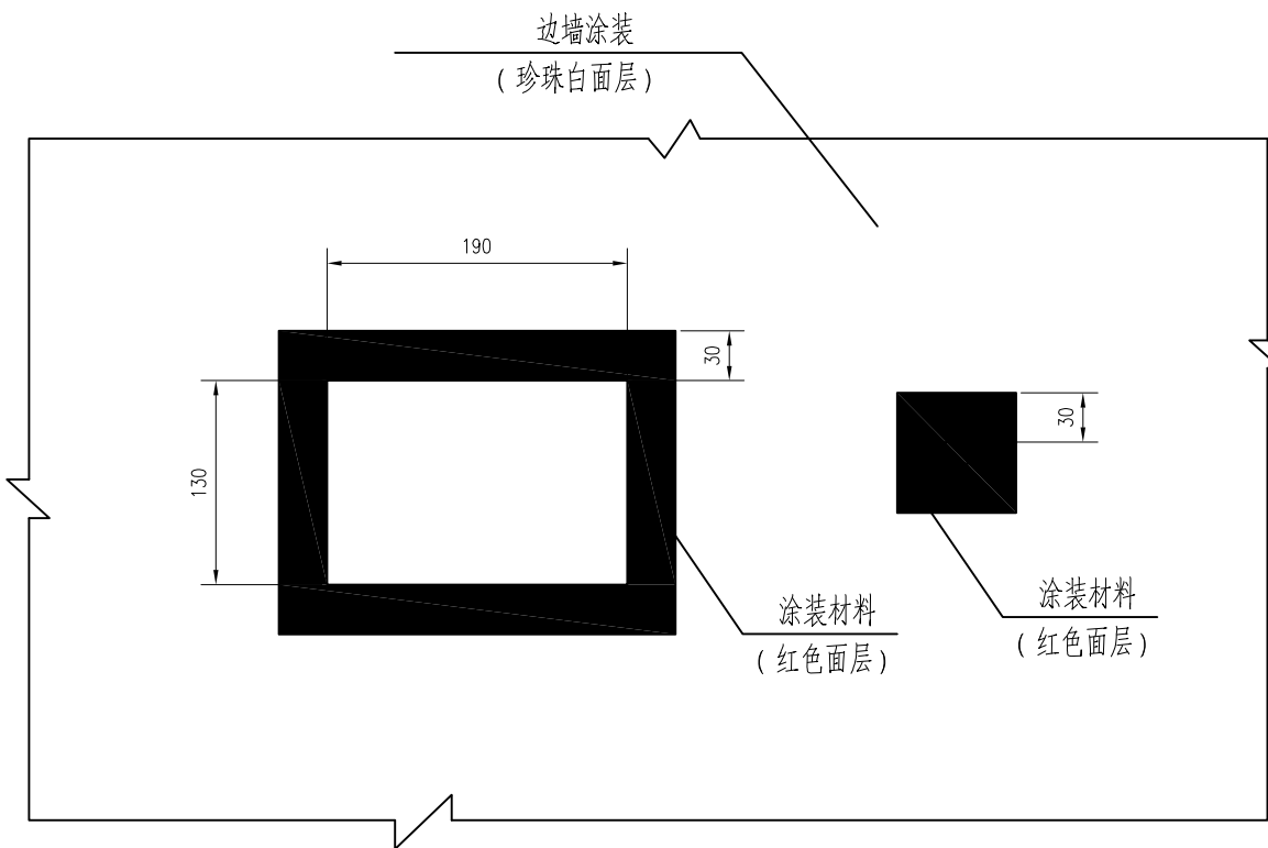
消防洞室I涂装立面图
