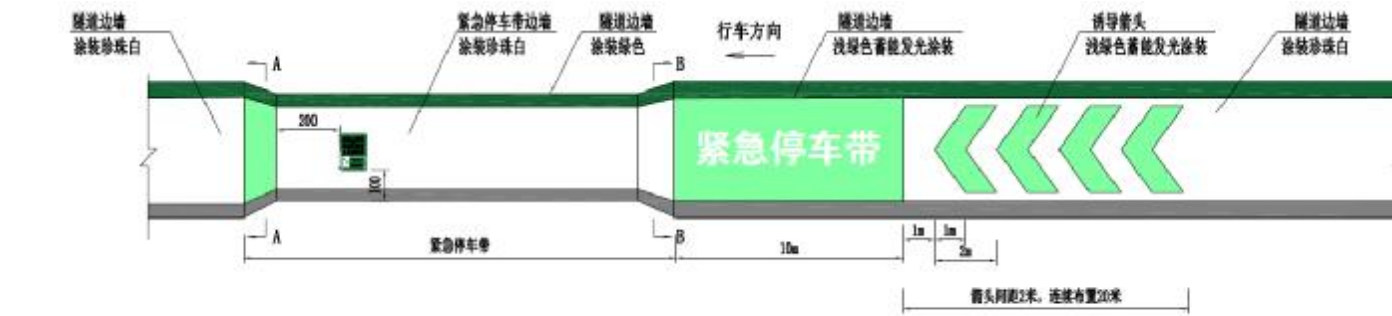
图 8 紧急停车带壁面标识设计
