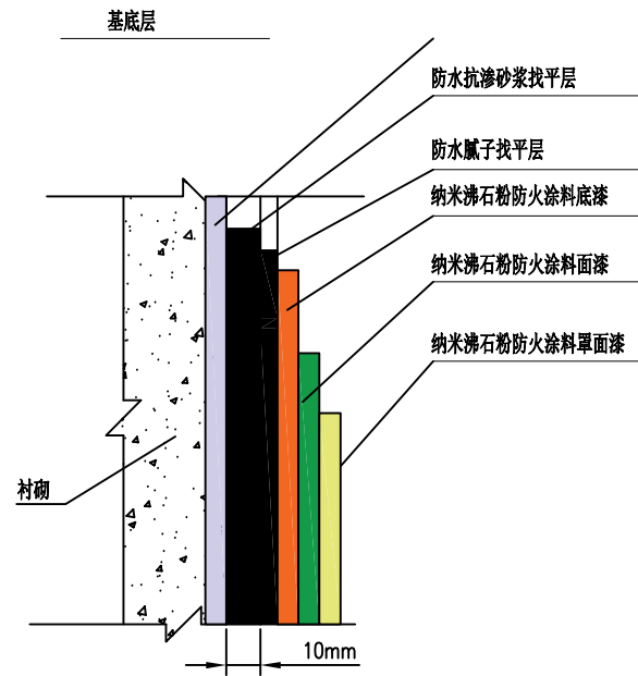
隧道壁涂料喷涂大样图
