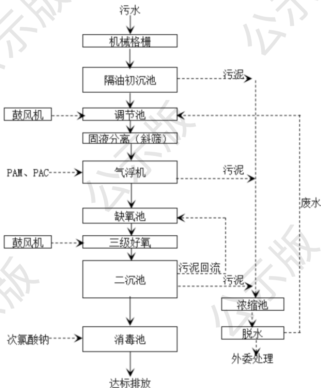
图7.2-2 废水处理工艺示意图
