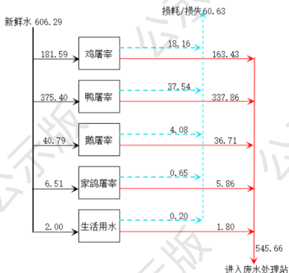
图 10.3-2 项目水平衡图 (m³/d)
