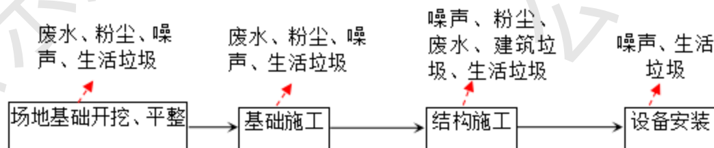
图 2.9-1 项目施工过程及产污环节示意图
