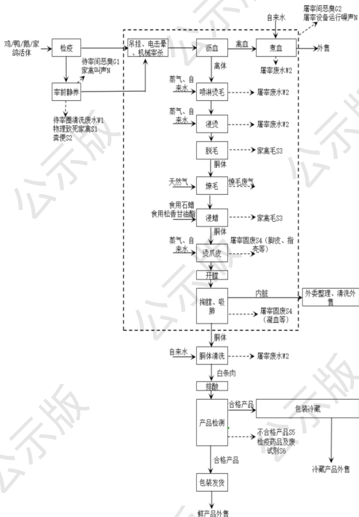
图 10.3-1 项目生产工艺及产排污环节示意图
