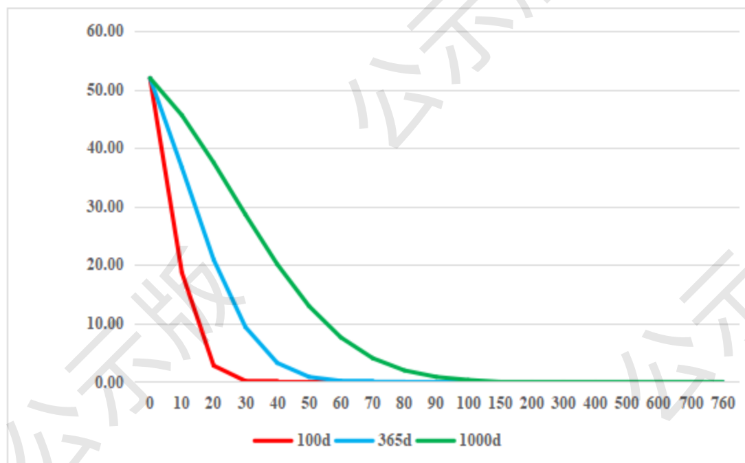
图 5.3-2 泄露点下游地下水中氨氮浓度情况
