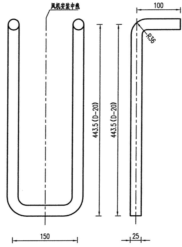
支座2钢筋弯钩 1:5
