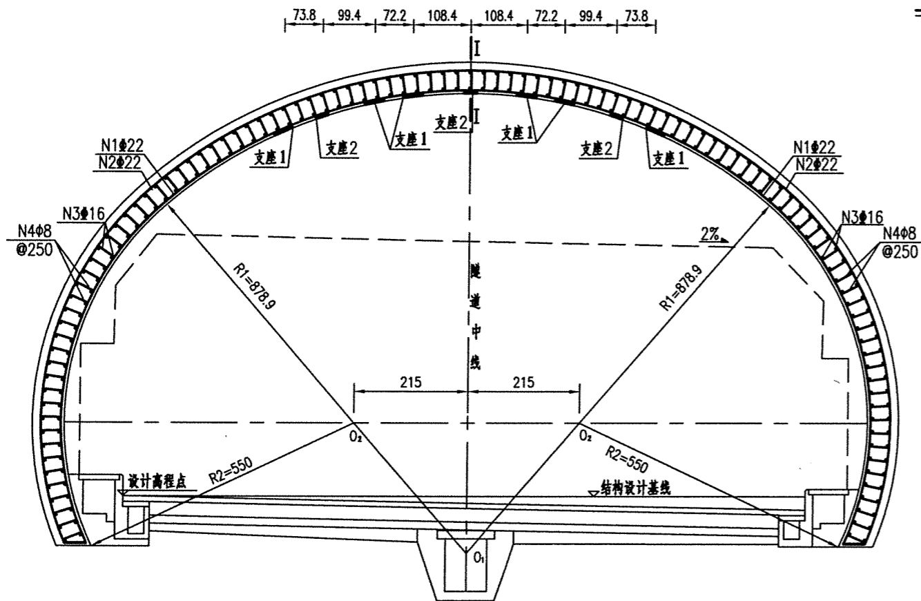
隧道射流风机悬挂段衬砌钢筋布置横断面图1:100 (正常段)
