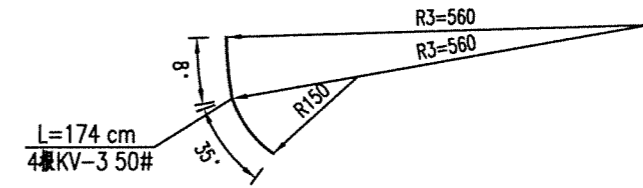
管1大样图 1:100
