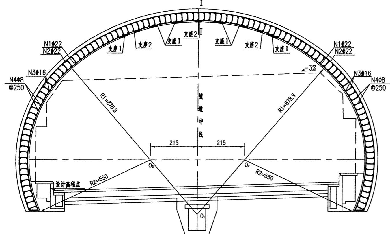
隧道射流风机悬挂段衬砌钢筋布置横断面图1:100 (反向超高段)
