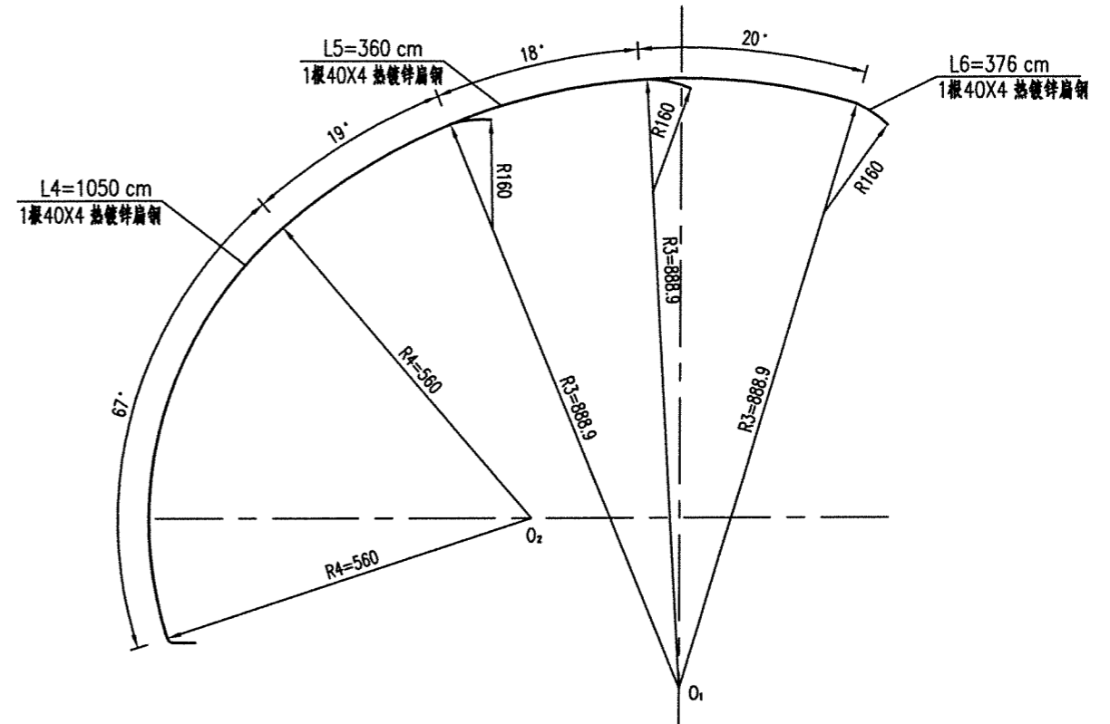
扁钢4、扁钢5、扁钢6大样图 1:100
