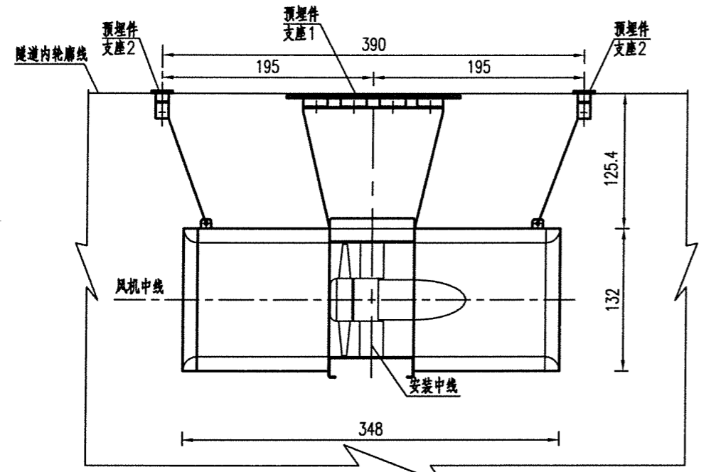
A-A剖面图 1:50
