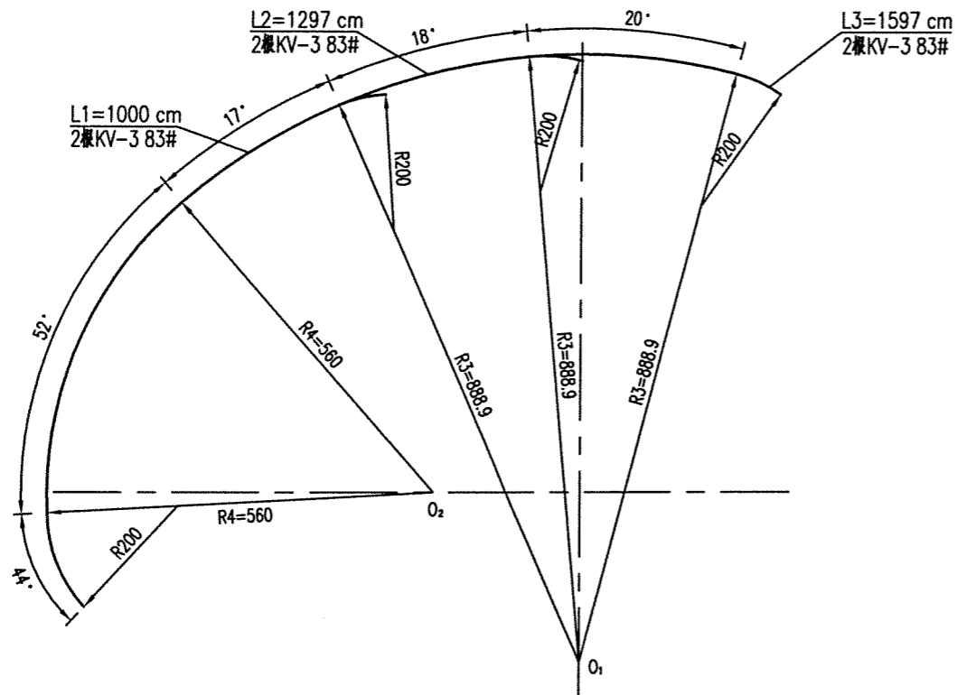
管1、管2、管3大样图 1:100
