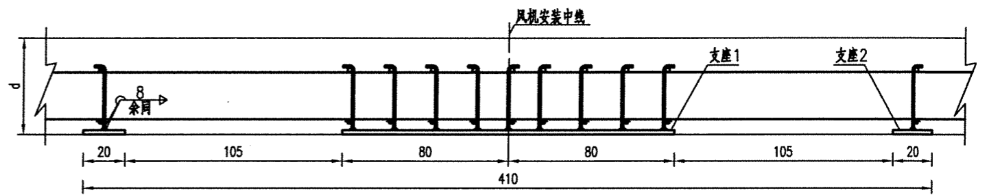
C-C剖面图 1:25
