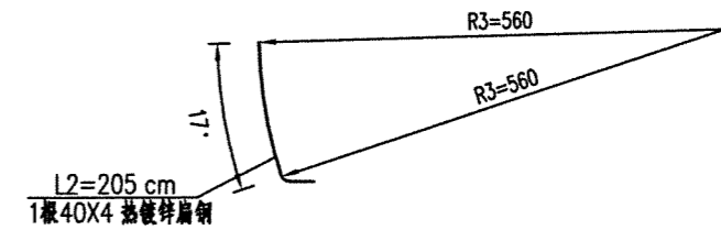
扁钢大样图 1:100
