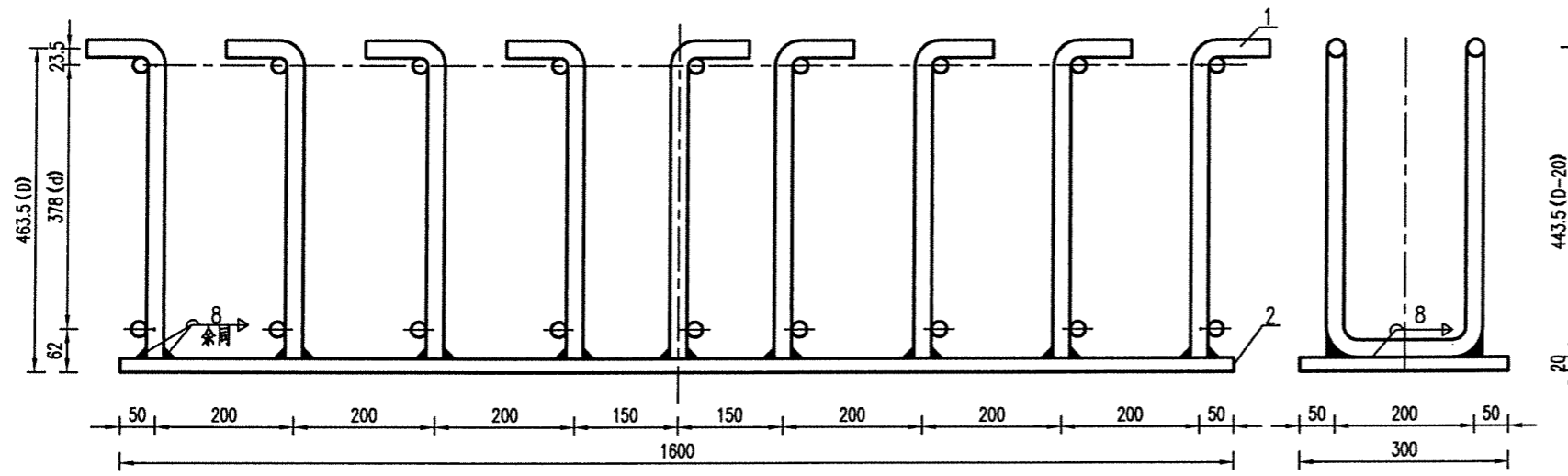
射流风机预埋件支座1 1:10
