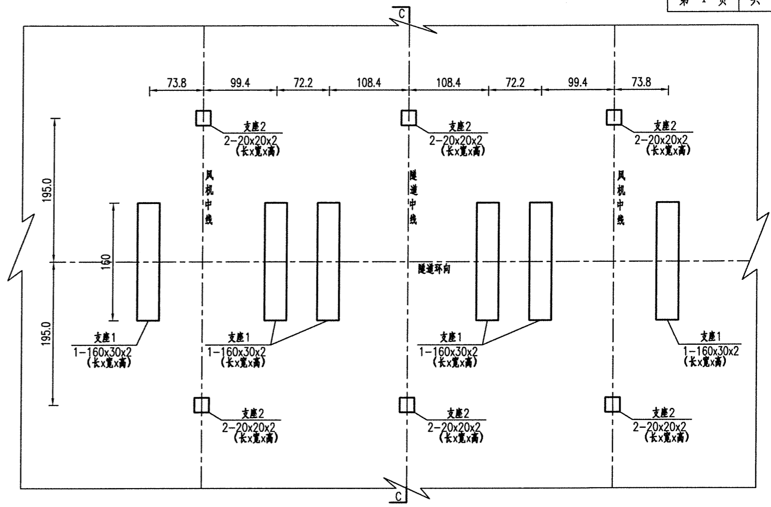
B-B剖面图 1:50
