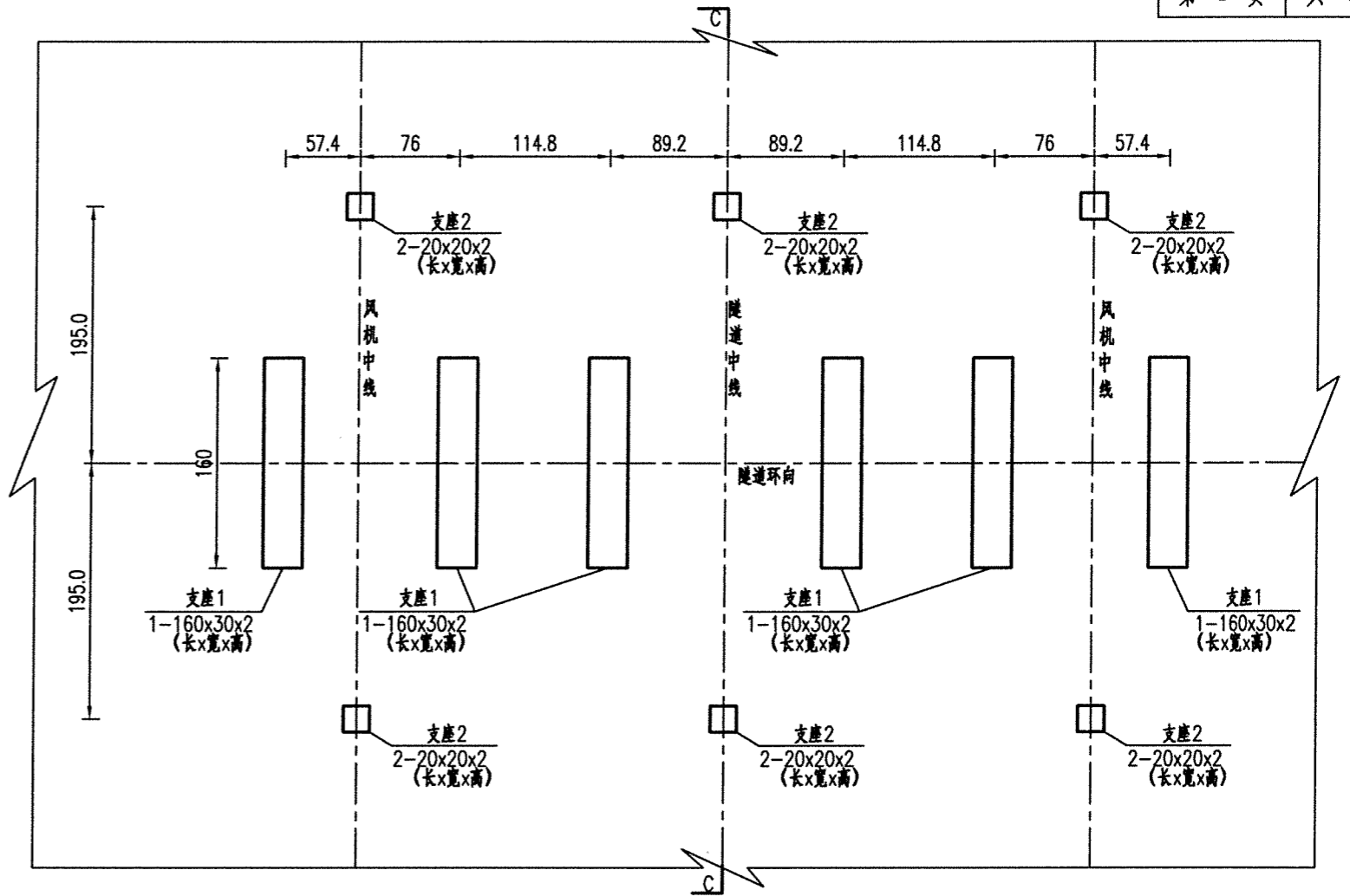
B-B剖面图 1:50
