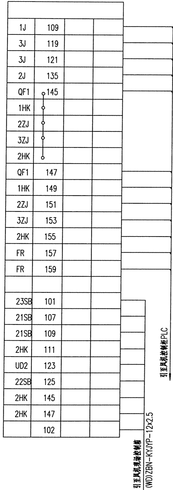
相应低压开关柜端子排接线图
