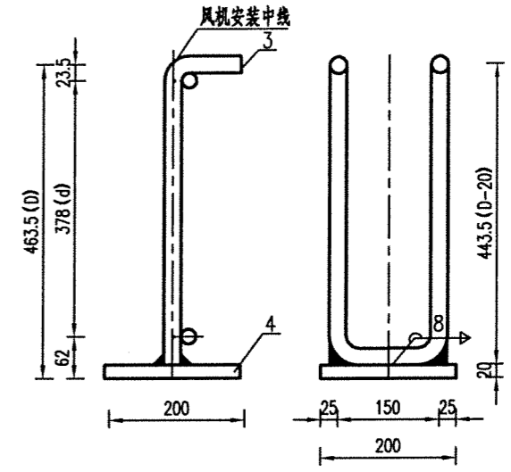
射流风机预埋件支座2 1:10
