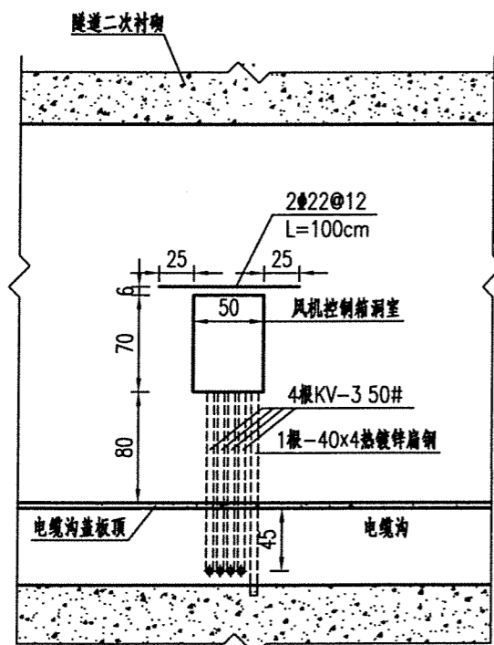
A-A 1:50
