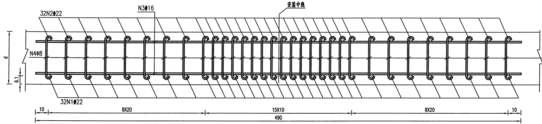
I-I 1:20
