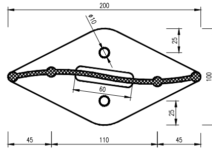
A-A 1: 2.5
