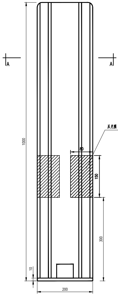
防眩板大样图 1: 5
