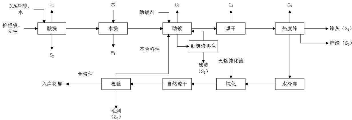
图 3.2-3 热镀锌工段工艺流程图
