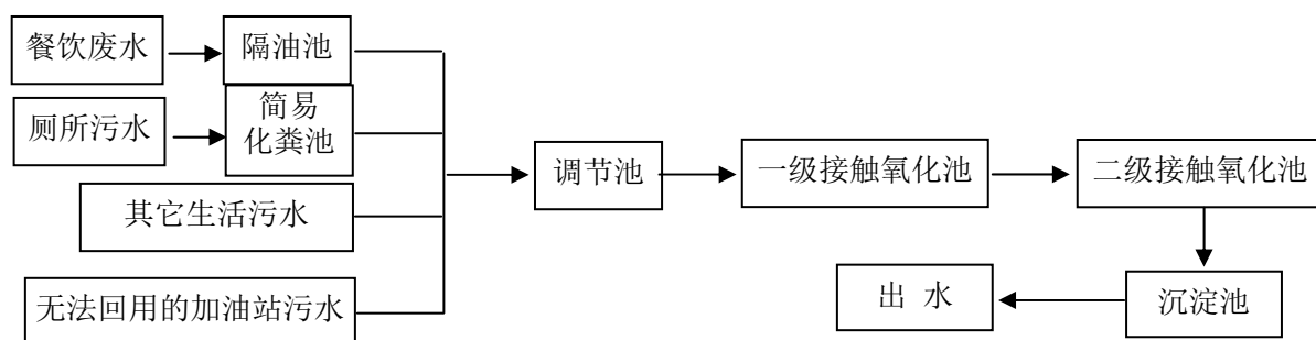
图 8.1.3-1 二级接触氧化法污水处理流程
