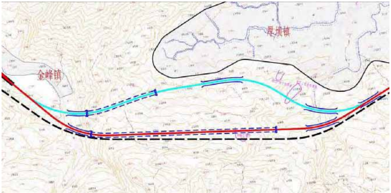
图 6.3-1 兴隆隧道段线布线示意图
