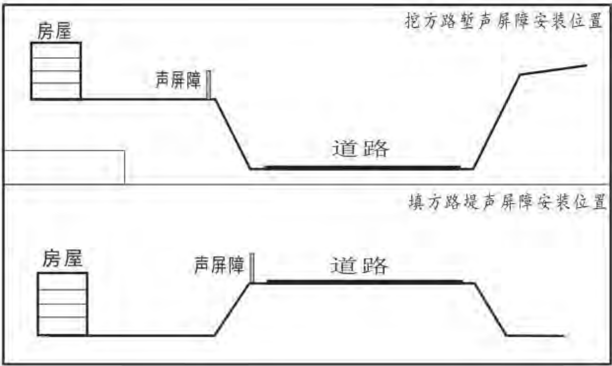
图 9.3.3-1 声屏障安装位置断面示意图
