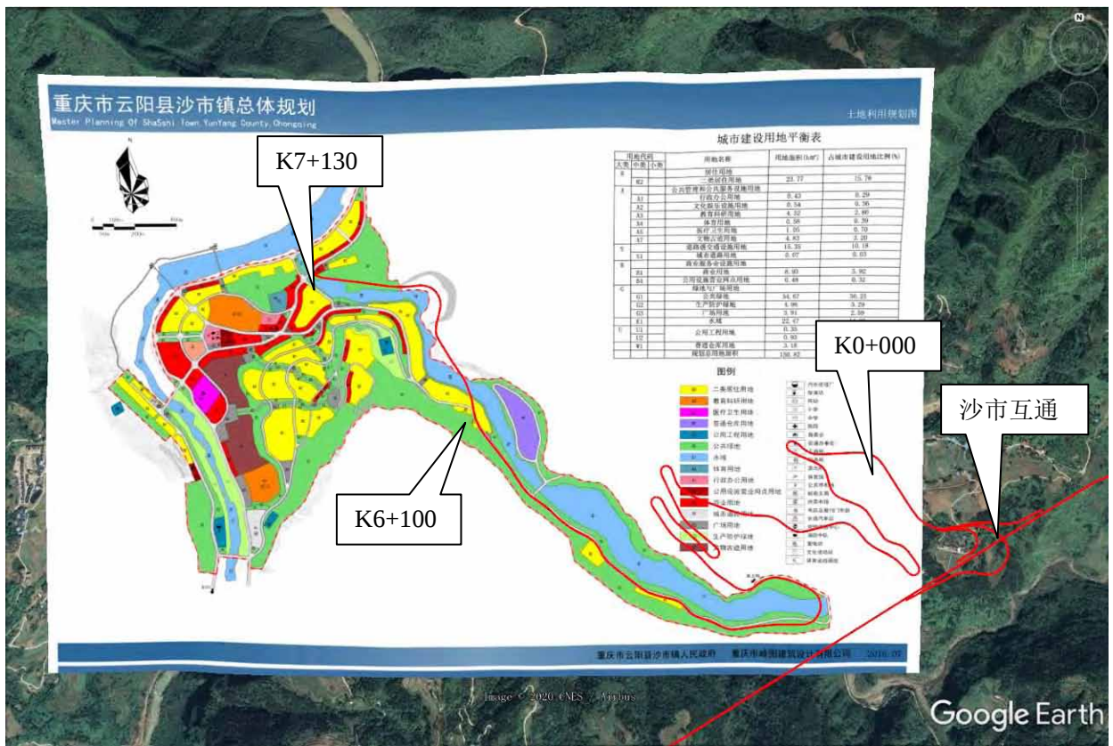
图 3.1.5-6 拟建公路与沙市镇规划位置关系图
