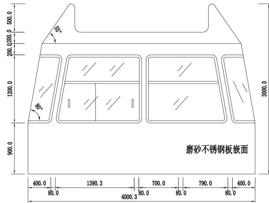
双人收费亭左侧大样图
