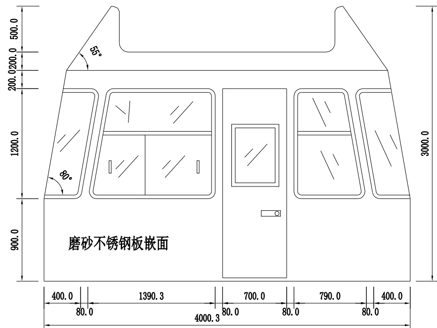
双人收费亭右侧大样图
