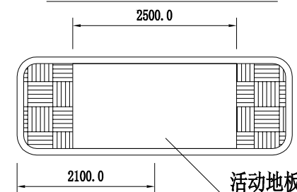
活动地板示意图1:80
