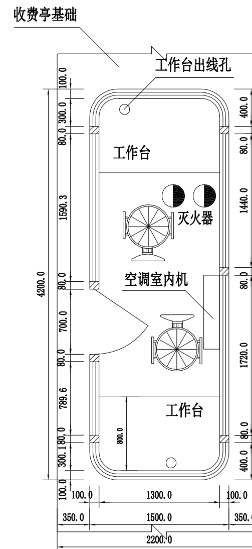
双人收费亭平面图
